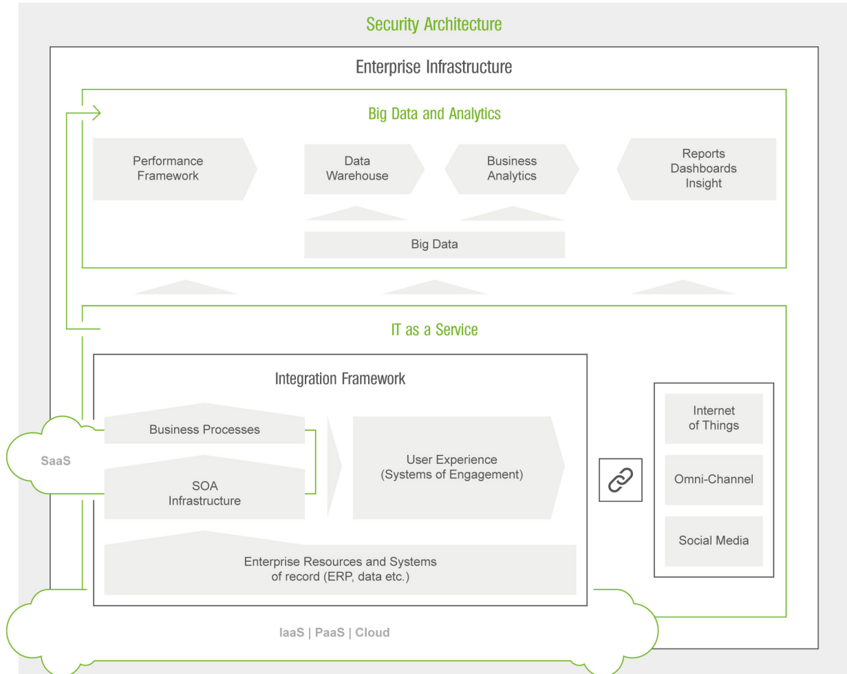
Abb.: Informationsarchitektur in der Digitalisierung
